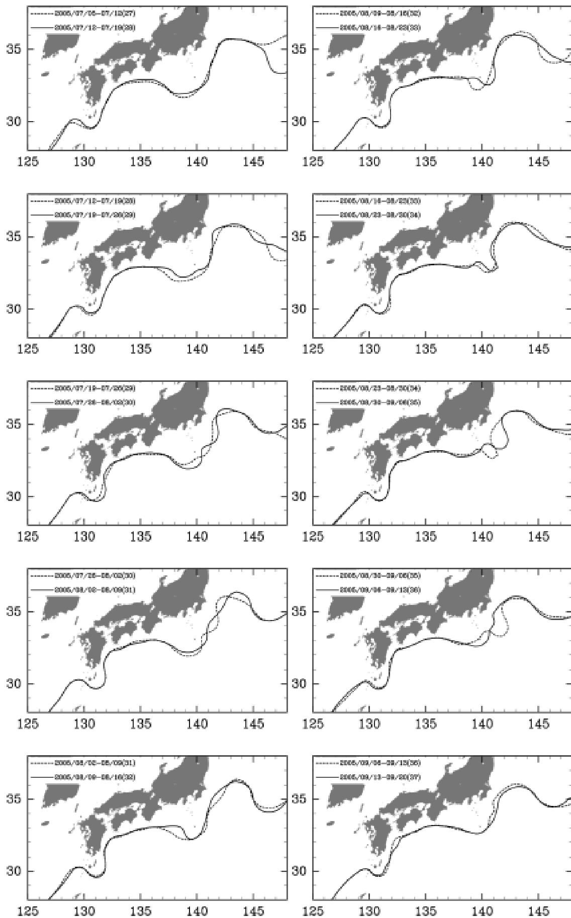
図 1 a 黒潮流軸のパターン
