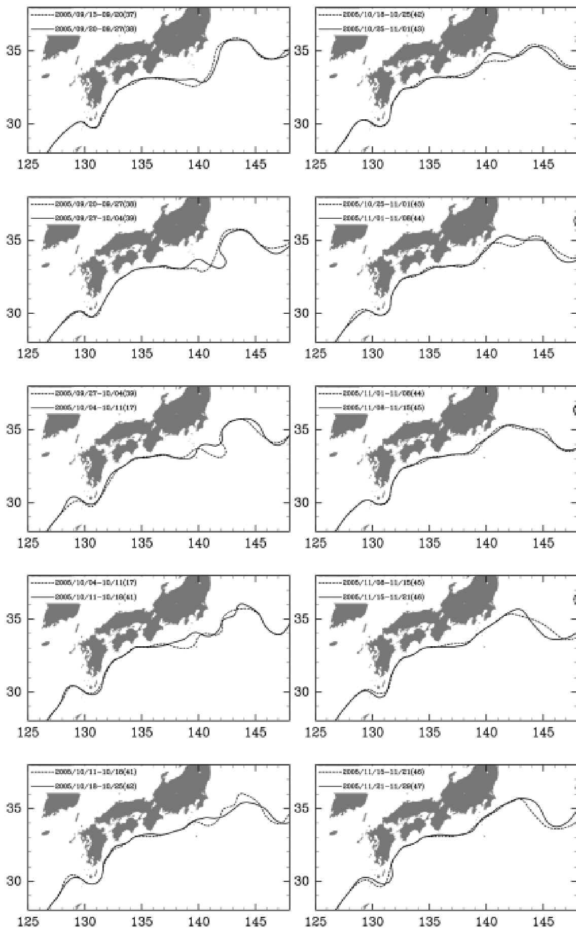
図 1 b 黒潮流軸のパターン
